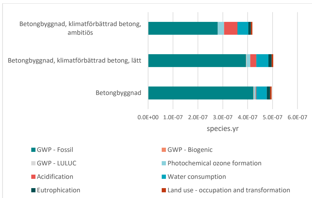
Figur 7: Betongdelarnas bidrag i betongscenarierna (per m² BTA). Den marginella reduktionen i GWP i 'lätt' vägs upp av högre potentiell påverkan av förorening och fotokemisk ozonbildning, i 'ambitiös' ger klimatförbättringen netto lägre påverkan.
